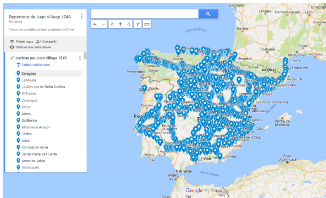
Figure 5. (Figura 5) Imagem do mapa dos núcleos representados na cartografia de Villuga de 1546 criado na plataforma do Google Engine.
