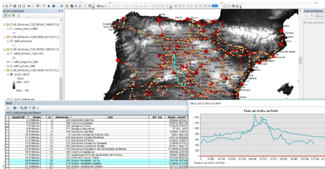
Figure 7. (Figura 7) Camada dos itinerários criada, sua tabela de atributos e cálculo do comprimento real de cada itinerário levando em consideração a topografia. Nesta imagem foram seleccionados os itinerários que iam de Toledo para Valladolid, um foi clasificado por Villuga para ser percorrido com carro e o outro com cavalo.
