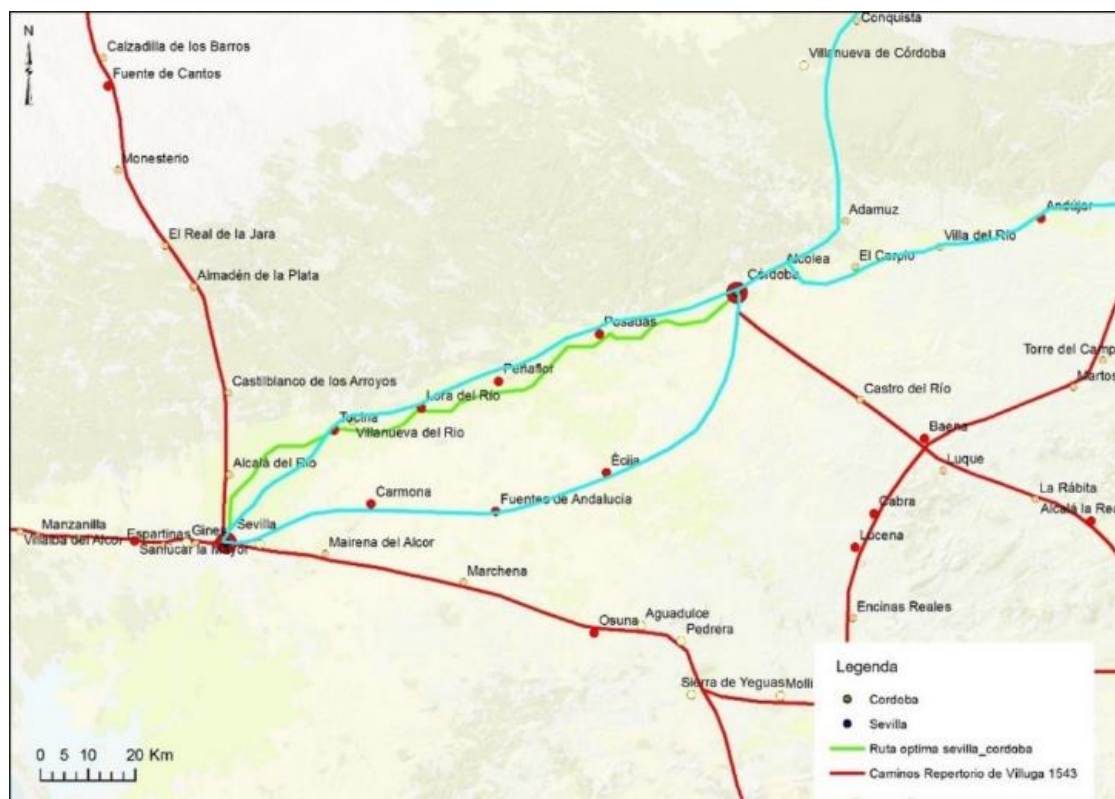
Figure 11. (Figura 11) Veja nesta imagem os itinerários 14 e 73 destacados em azul (Caves Barcelona - Sevilha e León-Sevilha, respectivamente) e o caminho de menor custo em verde.
